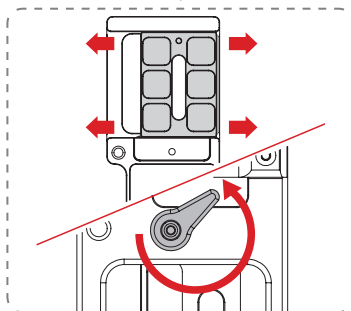
Пластина крепления
